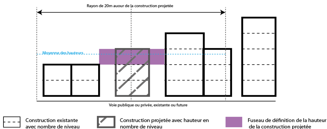
Schéma explicatif de définition de la hauteur des constructions
